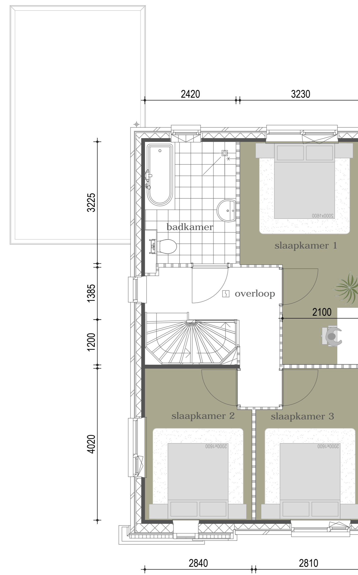
1e Verdieping
